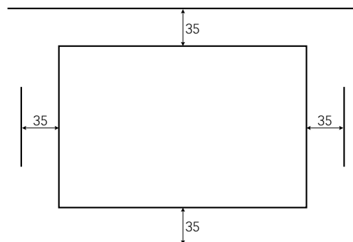
Distances minimales pour le montage (indications en mm)
